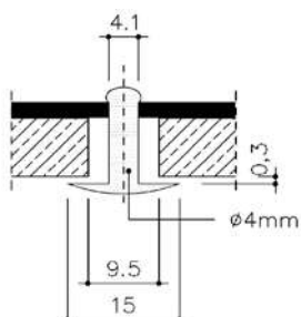
Vrij bevestigingspunt [G]
