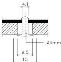
Vrij bevestigingspunt (G)
