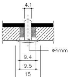
Vast bevestigingspunt (F)
