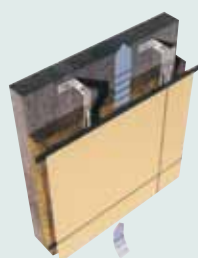
2. Zichtbare bevestiging op metalen draagstructuur
