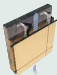
4. Onzichtbare bevestiging door middel van verlijming op metalen draagstructuur
