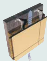
5. Onzichtbare bevestiging door middel van mechanische verankering op de rugzijde van de plaat (Tergo-systeem)
